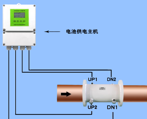
电池供电双声道超声波流量计（管段式）
